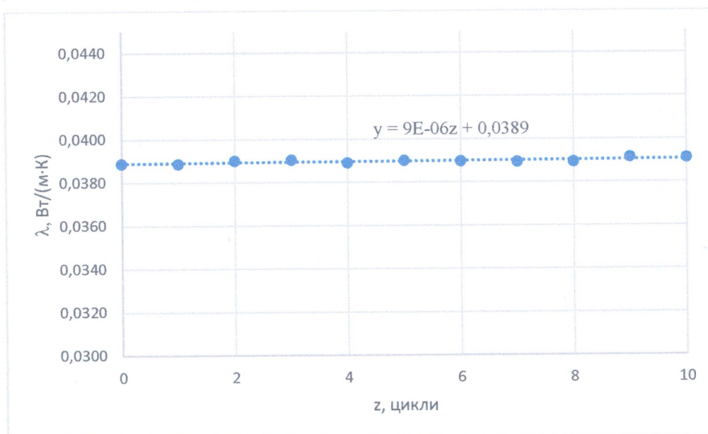
Рисунок 5 – Залежність теплопровідності від циклічних впливів
