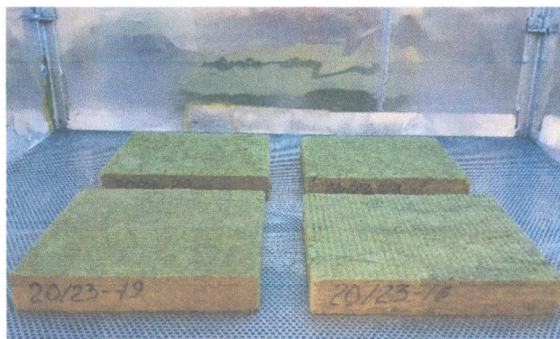
Рисунок 10 – Загальний вигляд дослідних зразків № 20/23 теплоізоляційного матеріалу марки «ТЕХНОФАС ЕФЕКТ» під час опромінення
