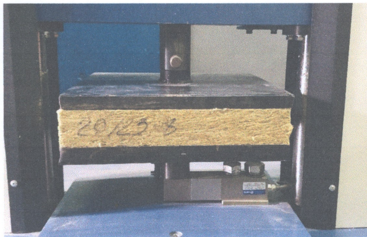
Рисунок 6 – Проведення випробування міцності на стиск при 10% деформації зразків № 20/23 теплоізоляційного матеріалу марки «ТЕХНОФАС ЕФЕКТ»
