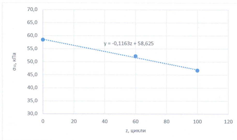
Рисунок 7 – Залежність міцності на стиск при 10% деформації від циклічних впливів зразків № 20/23 теплоізоляційного матеріалу марки «ТЕХНОФАС ЕФЕКТ»
