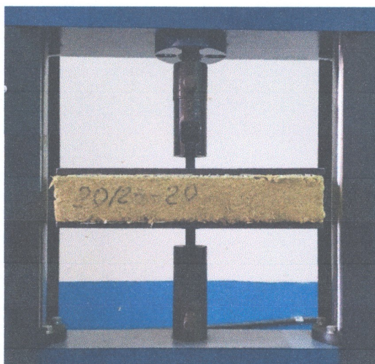
Рисунок 8 – Проведення випробування міцності при розтягу у напрямку, перпендикулярному до площини виробу зразків № 20/23 теплоізоляційного матеріалу марки «ТЕХНОФАС ЕФЕКТ»
