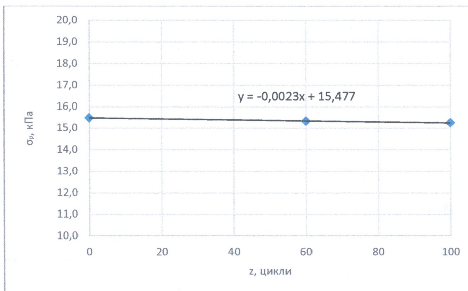
Рисунок 9 – Залежність міцності при розтягу у напрямку, перпендикулярному до площини виробу, від циклічних впливів зразків № 20/23 теплоізоляційного матеріалу марки «ТЕХНОФАС ЕФЕКТ»
